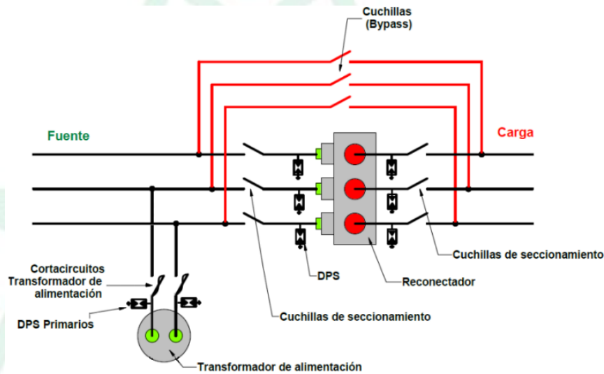
Figura 1. Esquema de conexión reconnector trifásico en troncal/ramal de más de 100A
