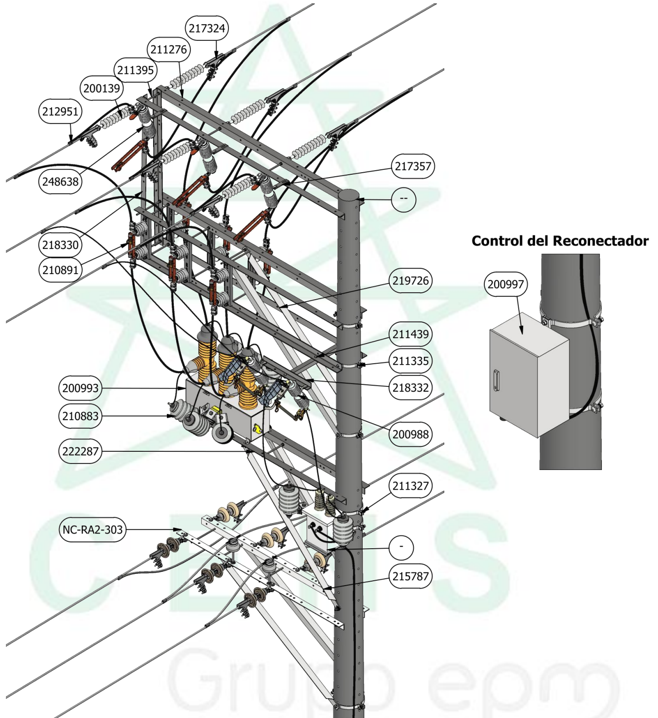
Figura 13. Detalle de montaje bandera doble nivel
