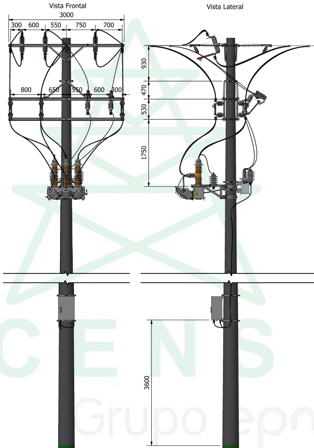
Figura 15. Dimensiones de montaje reconectador 34.5 kV horizontal
