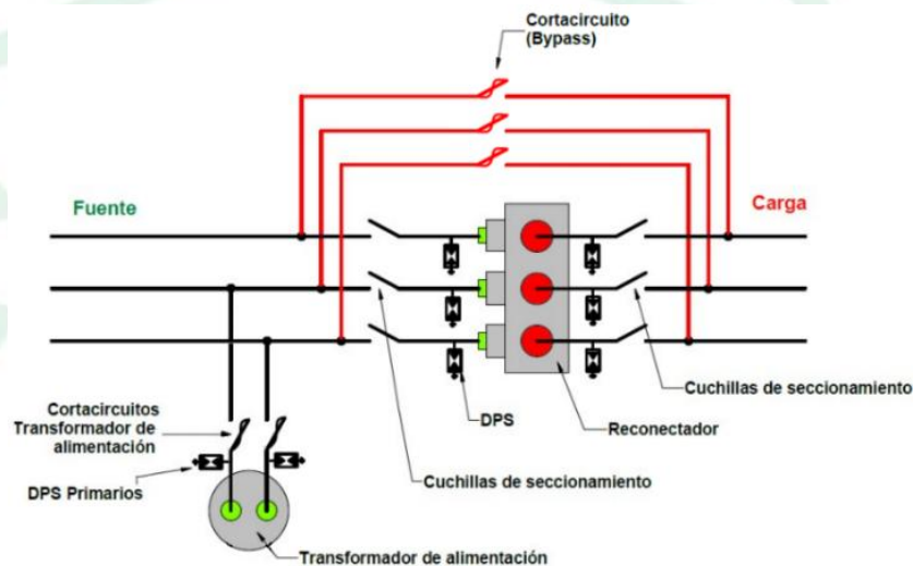
Figura 2. Esquema de conexión reconnector trifásico en ramal hasta 100 A
