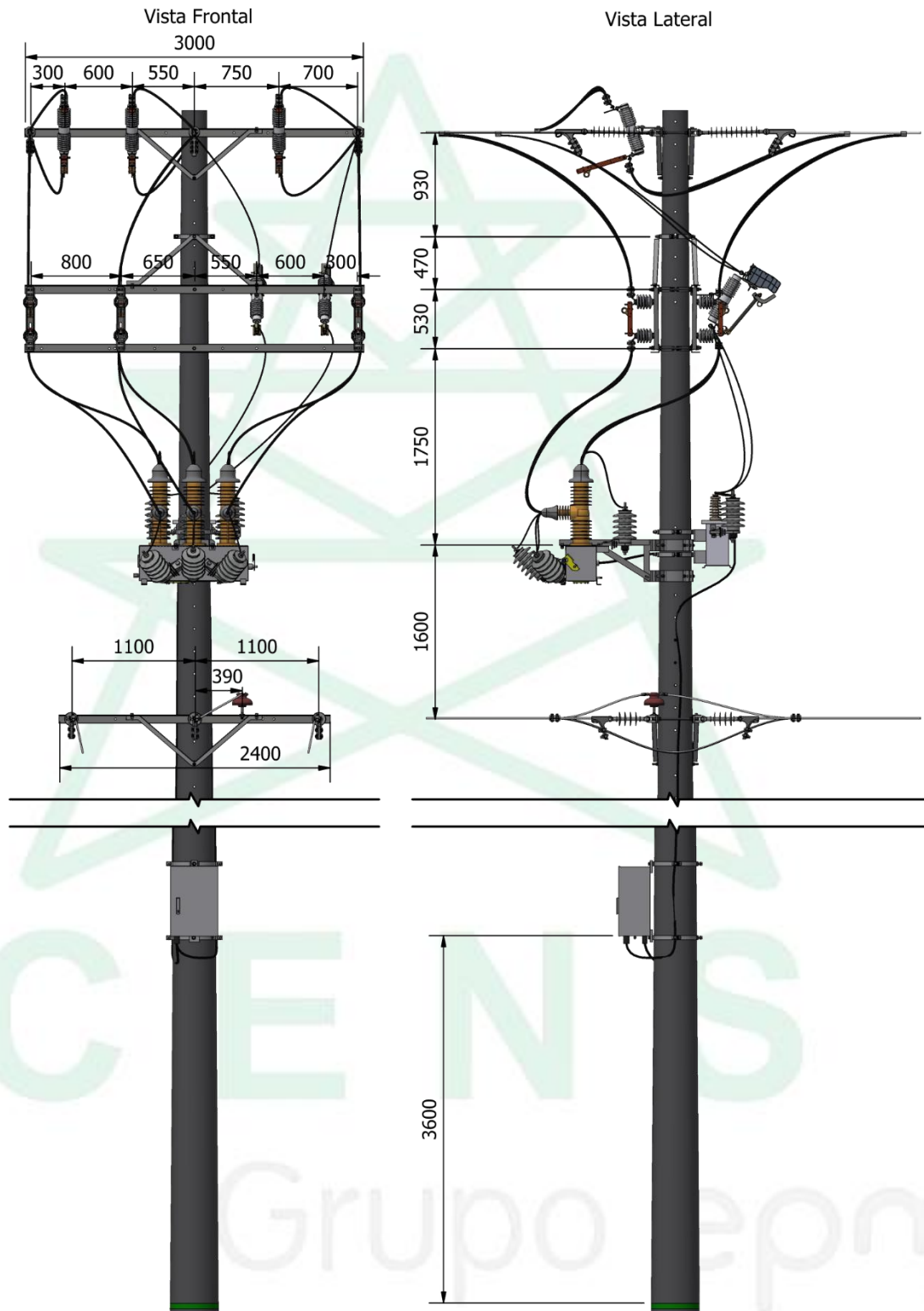
Figura 17. Dimensiones de montaje reconectador 34.5 kV horizontal doble nivel
