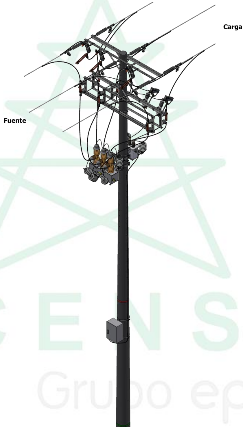
Figura 14. Vista isométrica
