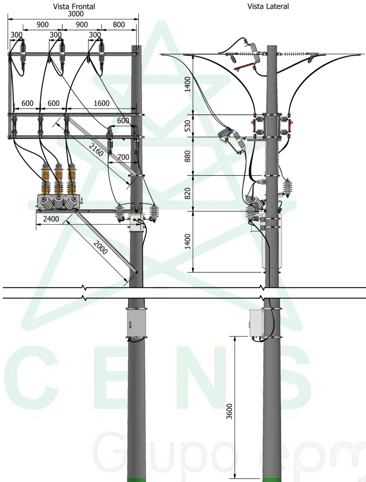
Figura 10. Dimensiones de montaje reconectador 34.5 kV - bandera
