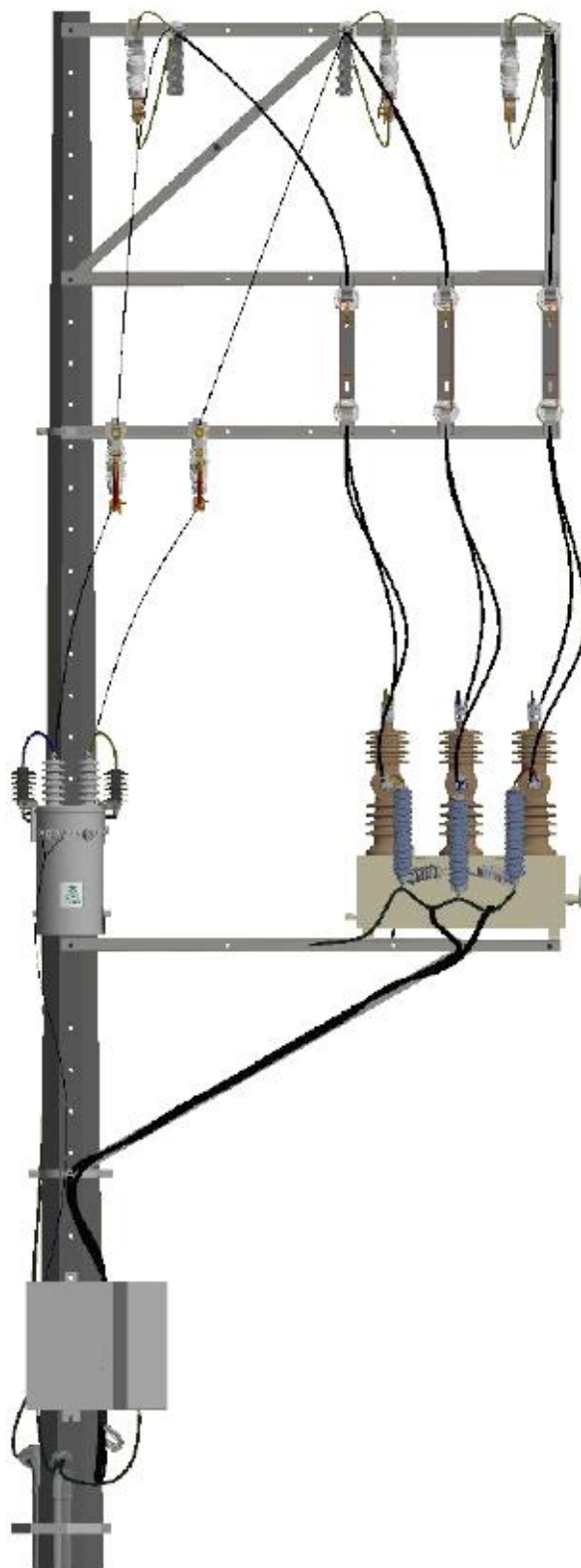
Figura 4. Esquema general del montaje del reconector 13.2kV– Vista de perfil
