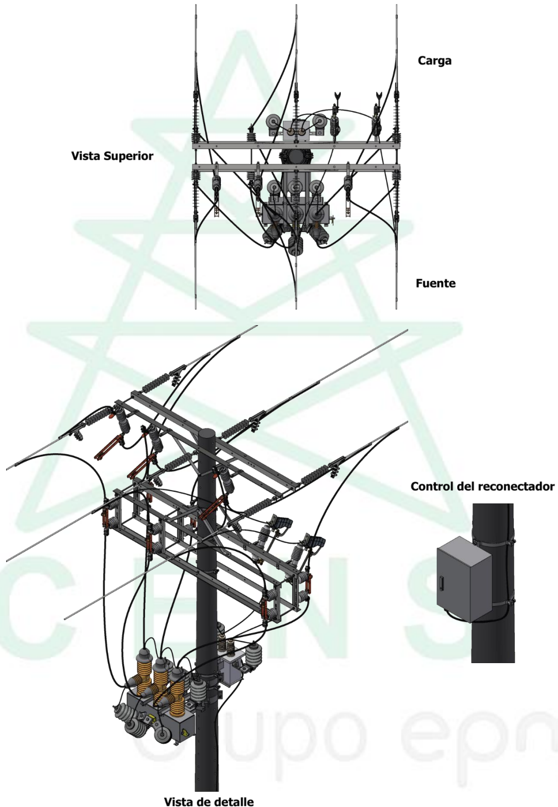
Figura 16. Detalle de montaje horizontal simple
