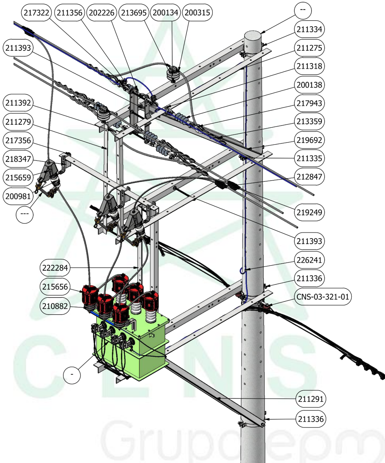
MONTAJE A: Detalle de materiales
