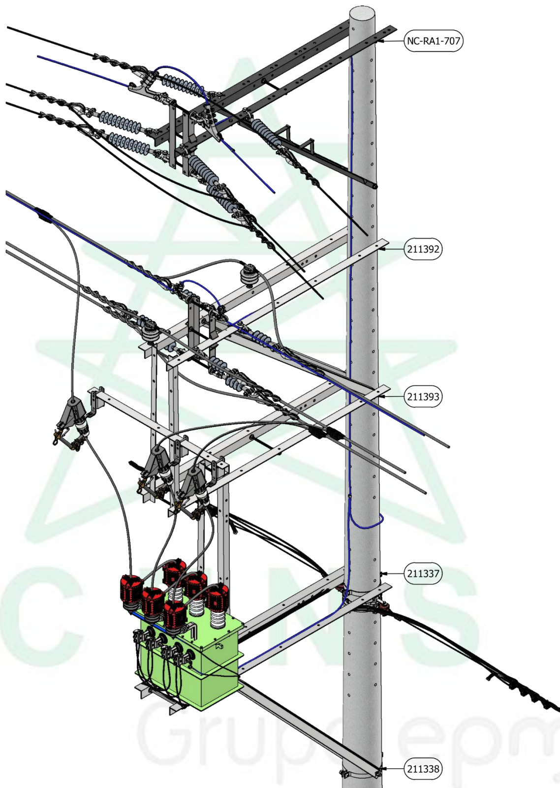
MONTAJE B: Detalle de materiales
