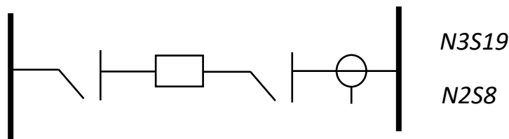
Figura 14. Diagrama Unifilar Bahía de acople – Convencional
