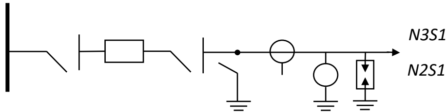
Figura 3. Diagrama Unifilar Bahía de línea - Barra sencilla - Convencional.
