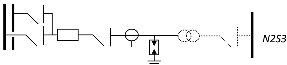
Figura 8. Diagrama Unifilar Bahía de transformador – Barra doble – Convencional Nivel 2
