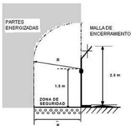
Figura 2. Distancias de seguridad contra contactos directos.
