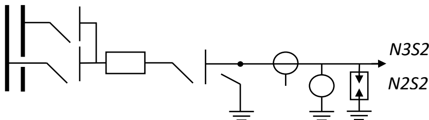
Figura 6. Diagrama Unifilar Bahía de línea – Barra doble - Convencional
