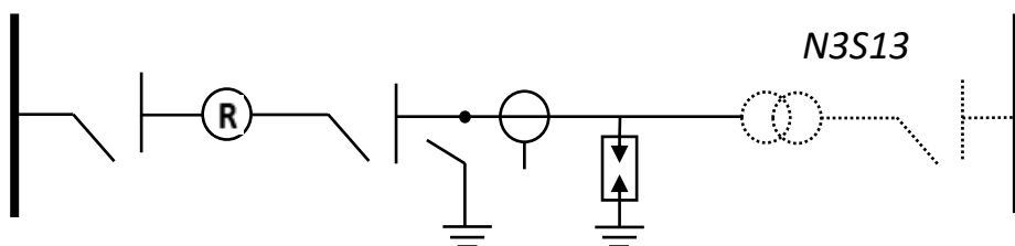
Figura 13. Diagrama Unifilar Bahía de llegada o salida – Subestación convencional reducida Nivel 3
