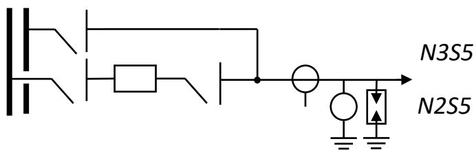
Figura 9. Diagrama Unifilar Bahía de línea – Barra principal y transferencia – Convencional
