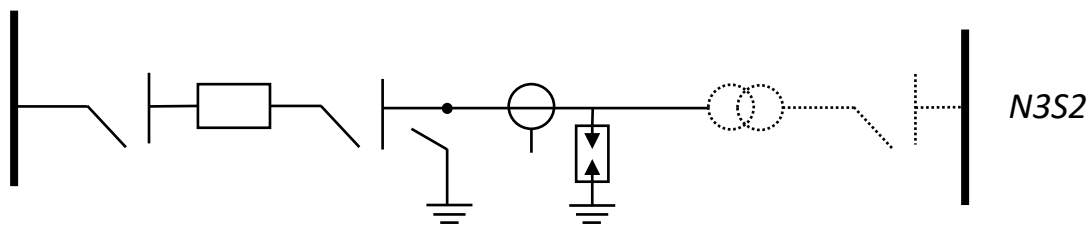
Figura 4. Diagrama Unifilar Bahía de transformador – Barra sencilla – Convencional Nivel 3
