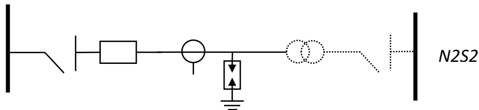
Figura 5. Diagrama Unifilar Bahía de transformador – Barra sencilla – Convencional Nivel 2
