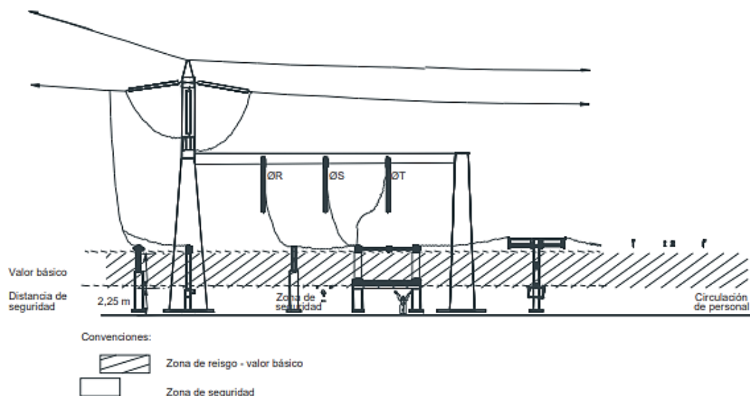
Figura 15. Zona de seguridad para circulación de personal
