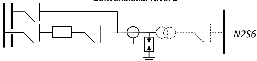
Figura 10. Diagrama Unifilar Bahía de transformador – Barra principal y transferencia – Convencional Nivel 3
