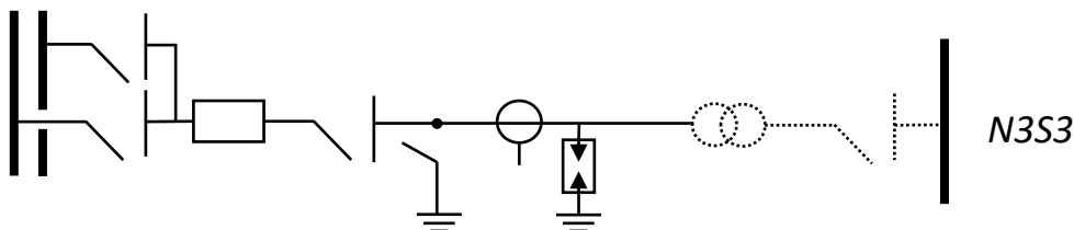
Figura 7. Diagrama Unifilar Bahía de transformador – Barra doble – Convencional Nivel 3
