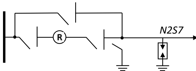
Figura 12. Diagrama Unifilar Bahía de línea – Subestación reducida Nivel 2
