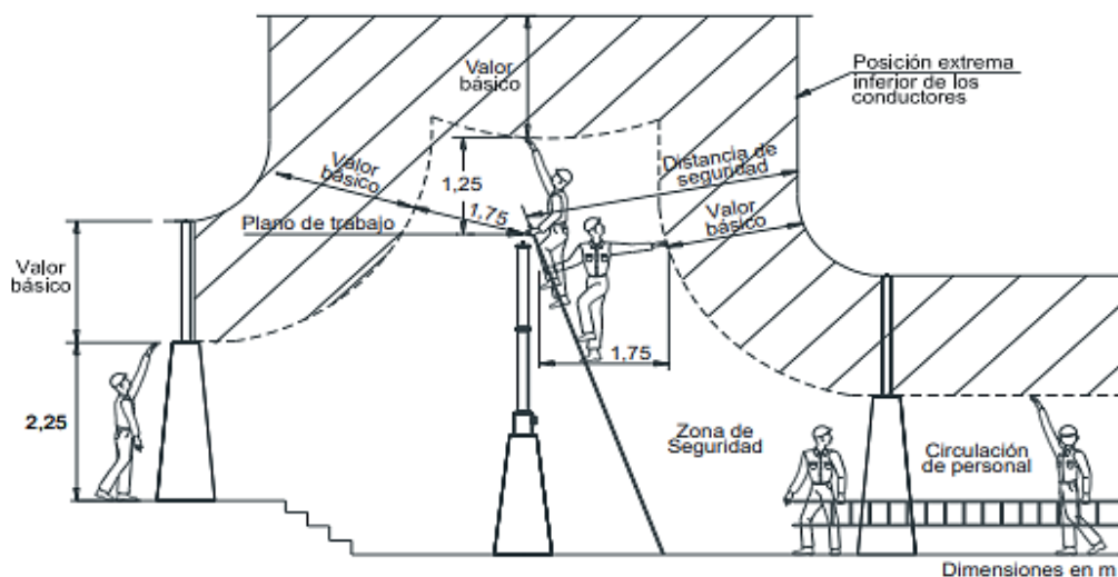
Figura 16. Zonas de seguridad
