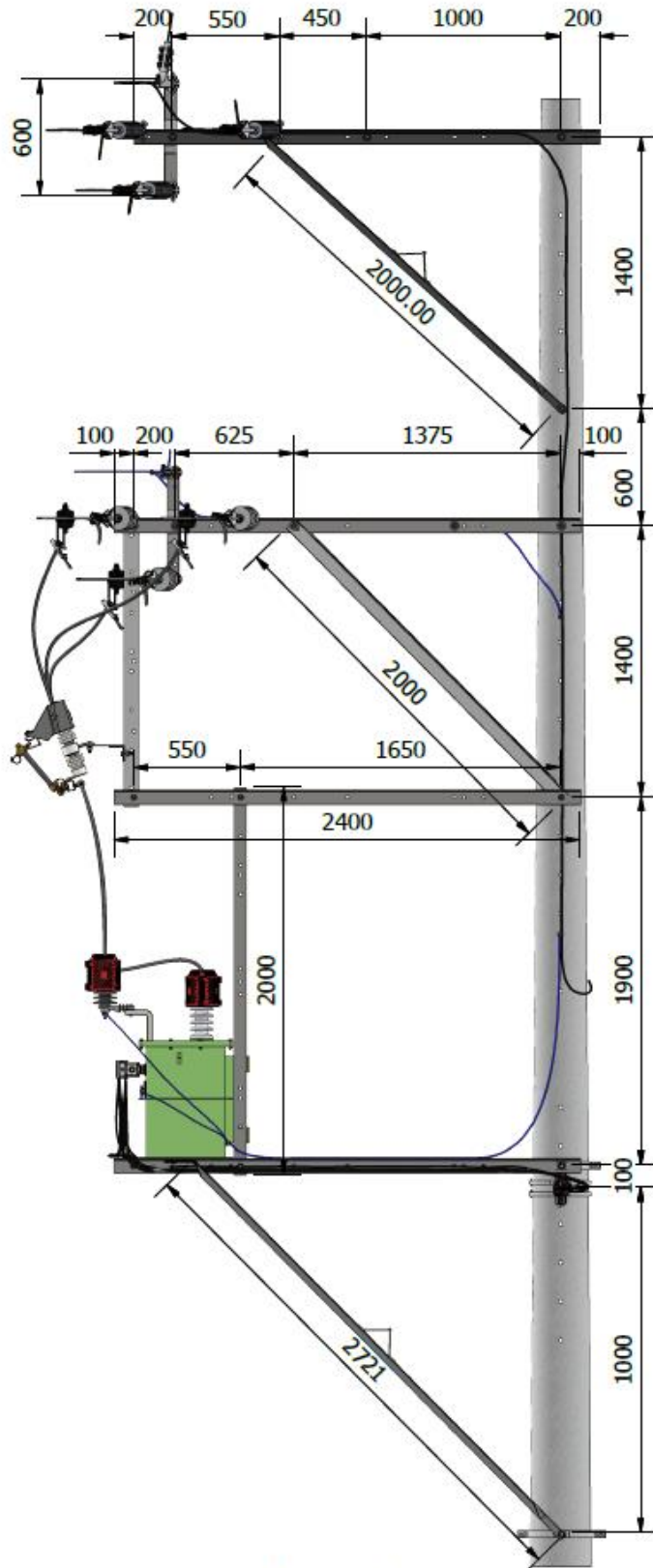
Vista lateral
