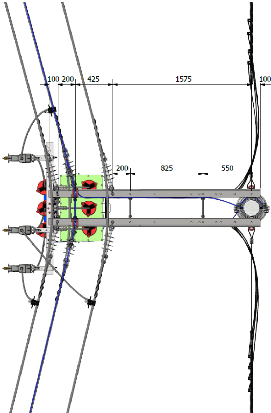
Vista Superior
