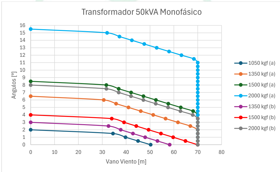
Figura 9. Curva de utilización transformador Monofásico de 50kVA
