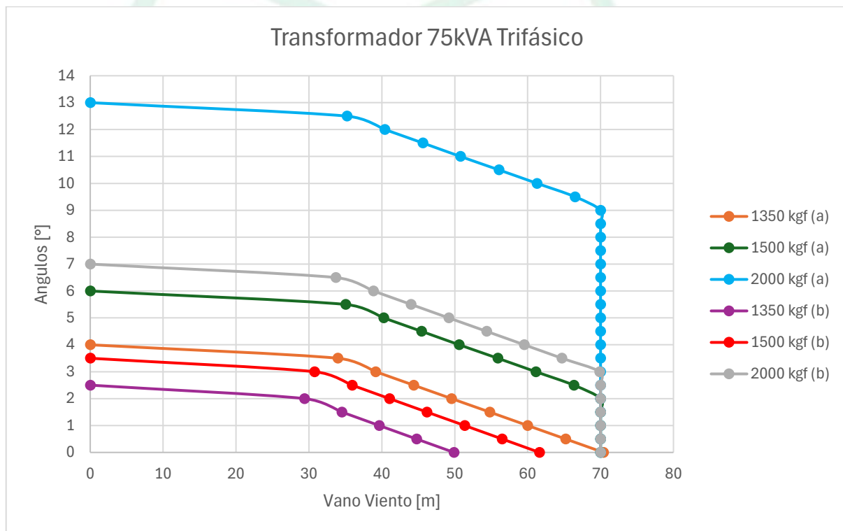
Figura 11. Curva de utilización transformador trifásico de 75kVA
