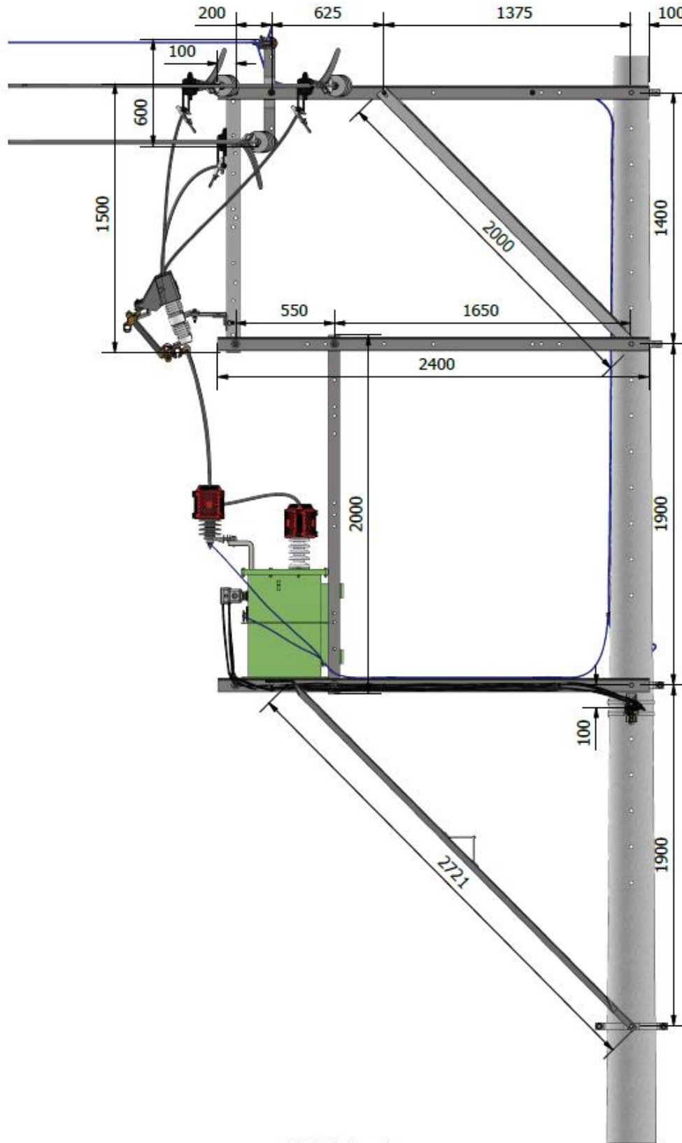
Vista Lateral
