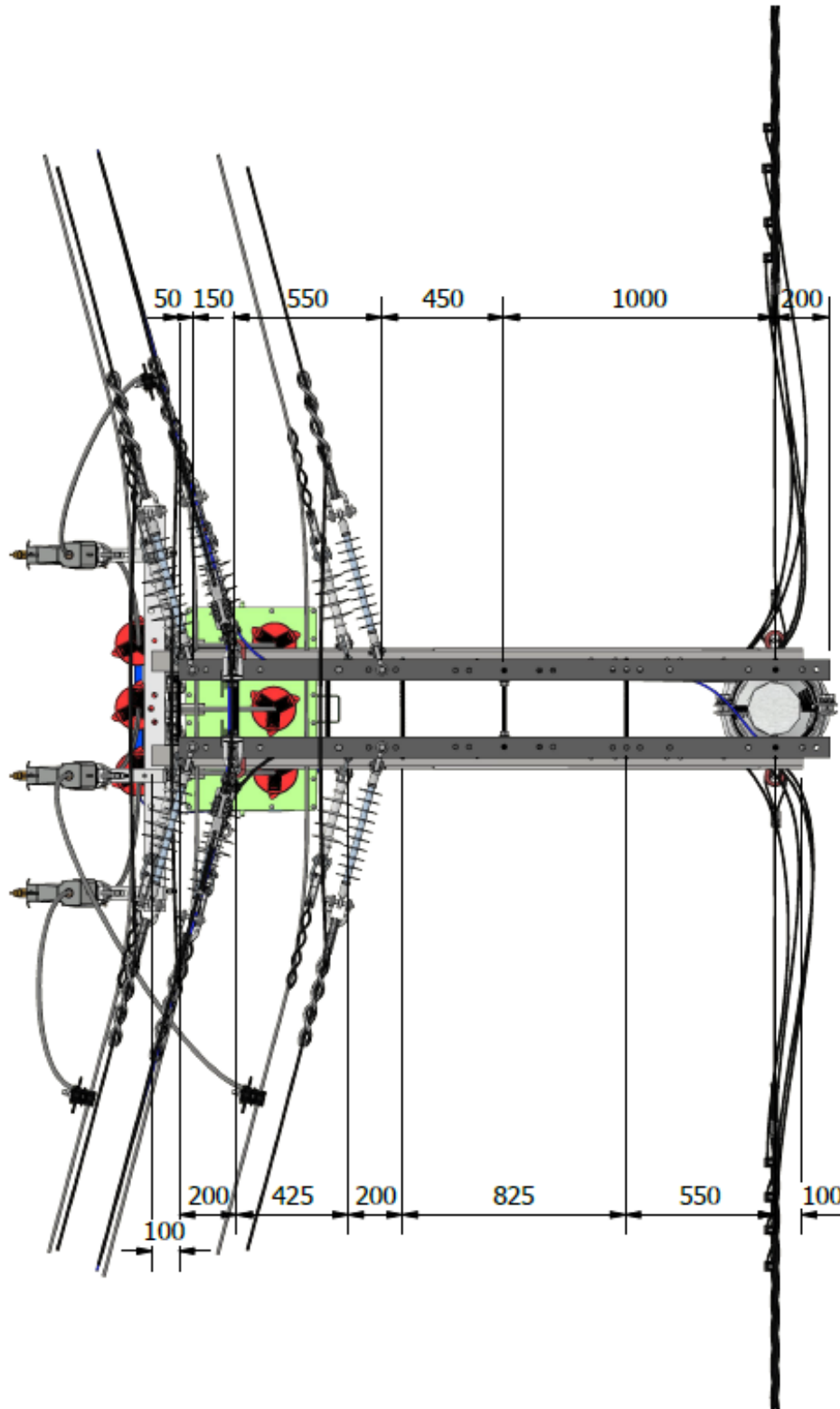
Vista superior
