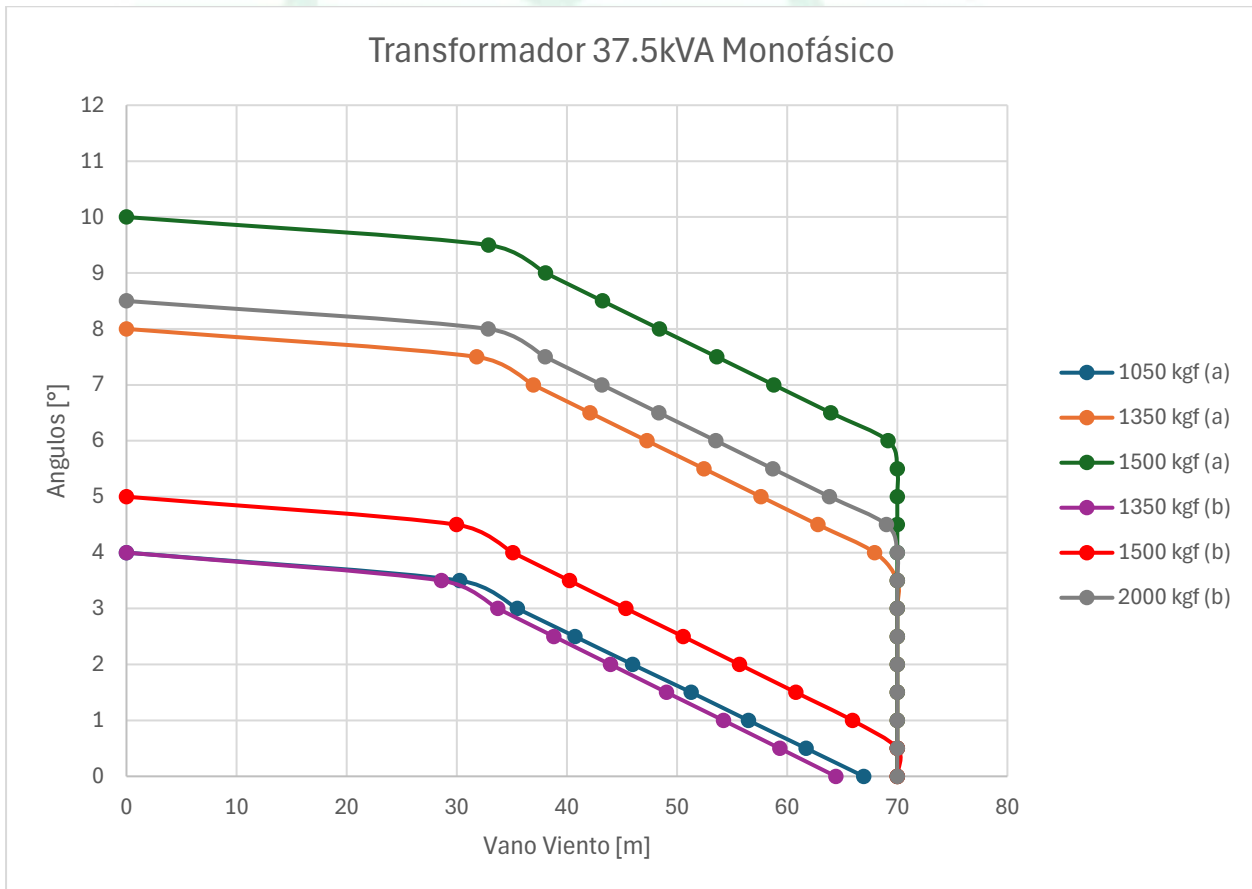
Figura 7. Curva de utilización transformador monofásico de 37.5kVA
