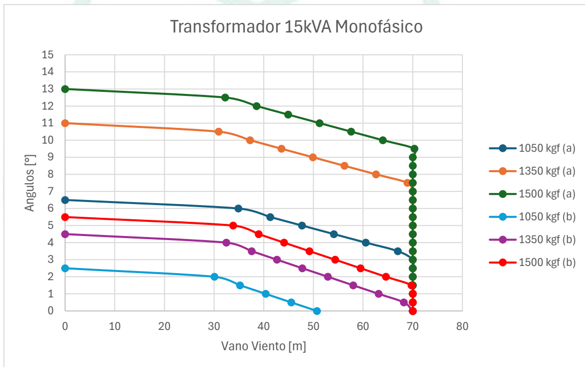
Figura 3. Curva de utilización transformador monofásico de 15kVA
