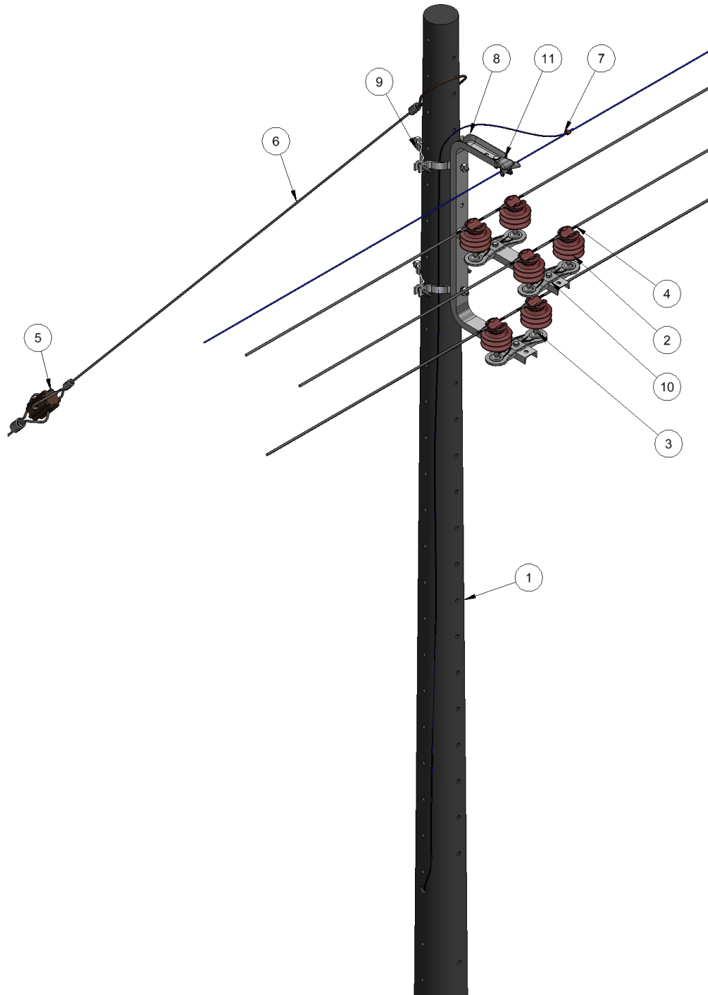
Figura 1. Vista isometrica.
