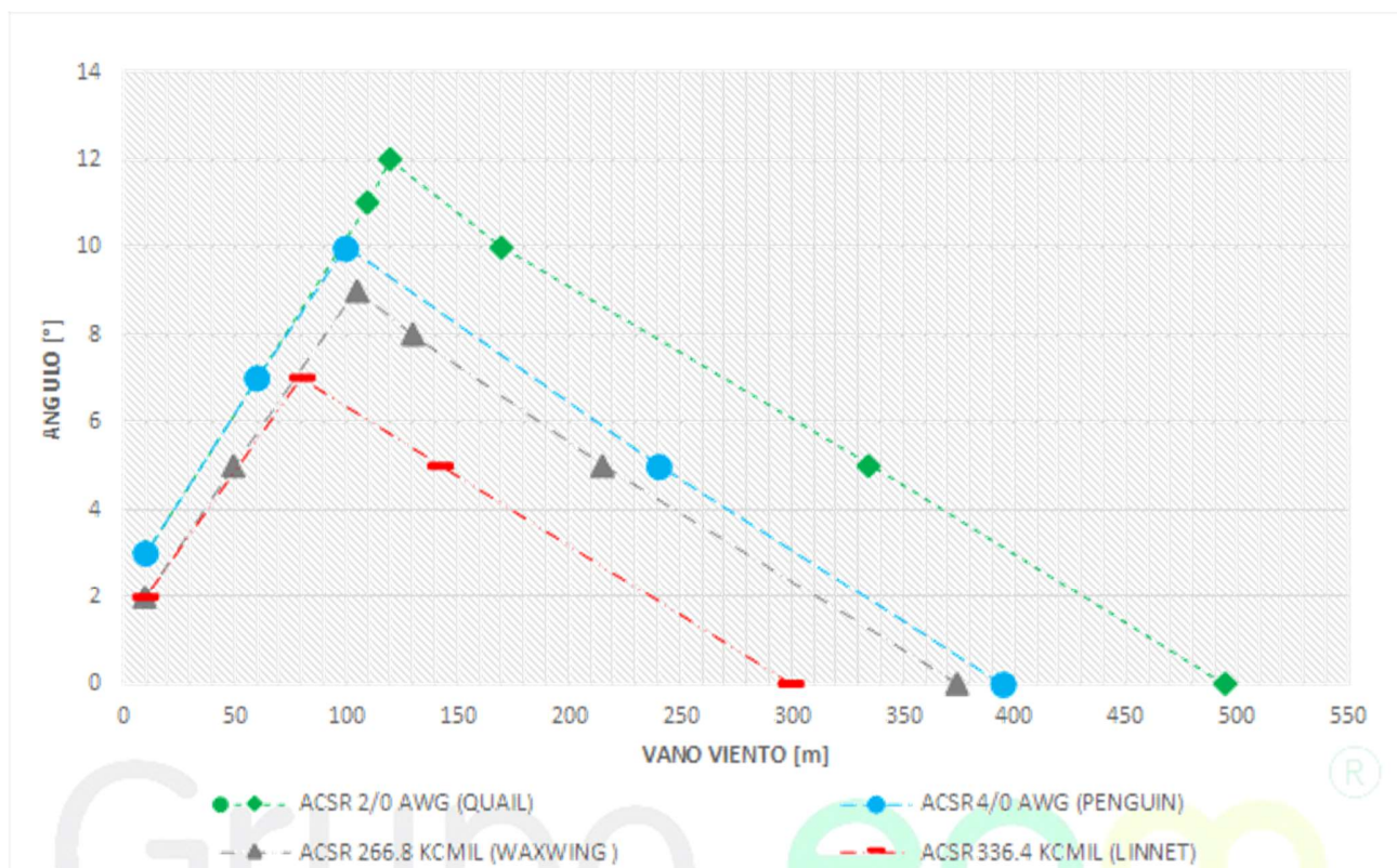
Figura 5. Curva de utilización para opción de montaje d: sin retenida y con bayoneta para soportar el cable de guarda/neutro
