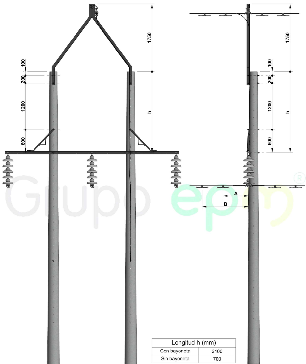
Figura 2. Vista frontal
