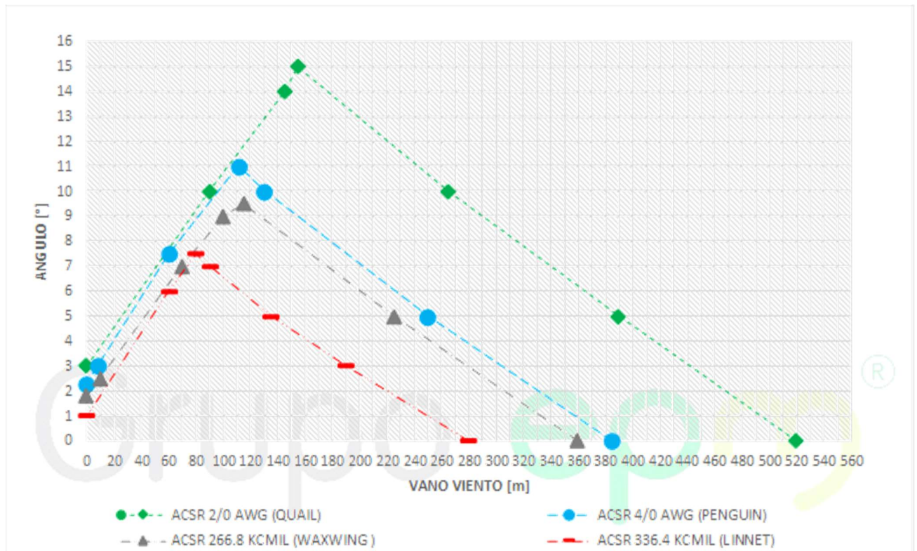
Figura 4. Curva de utilización para opción de montaje c: sin retenida y sin bayoneta
