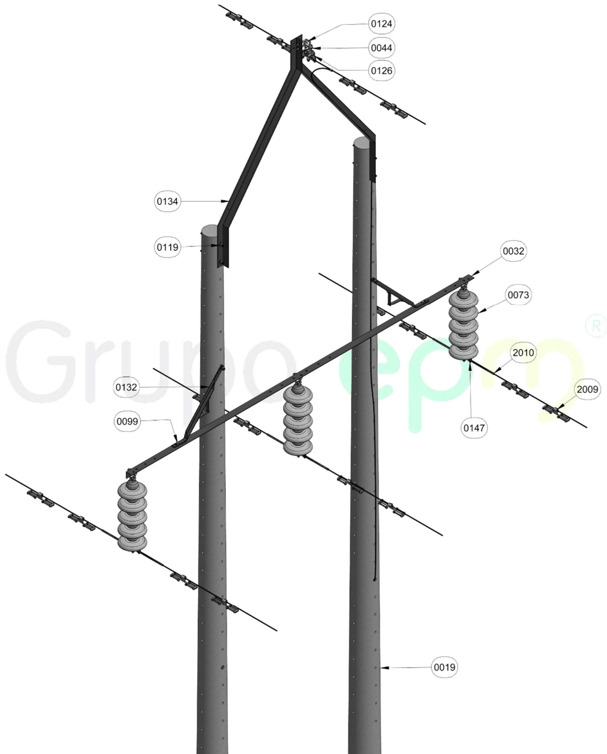
Figura 1. Vista isométrica
