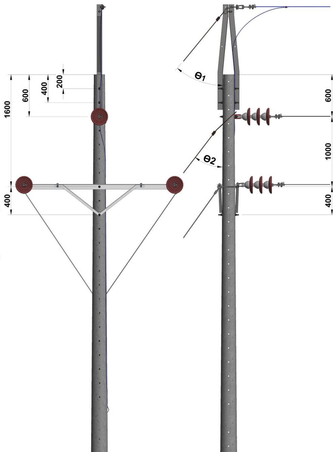
Figura 2. Vista frontal.
