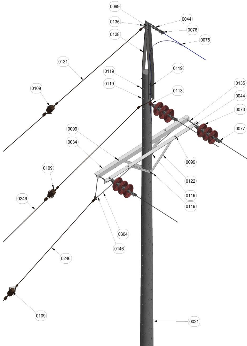
Figura 1. Vista isometrica.
