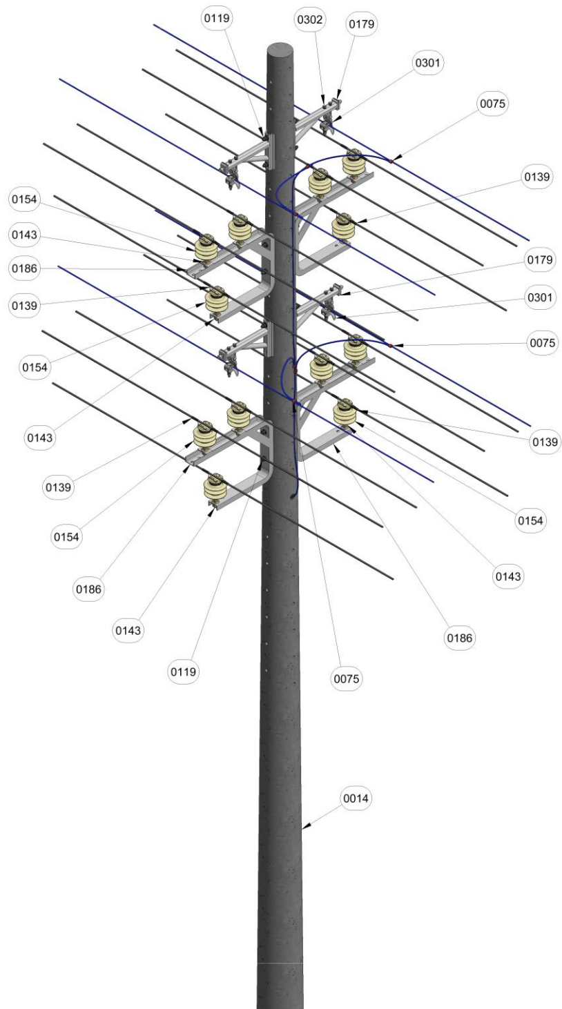
Figura 1. Vista isometrica.
