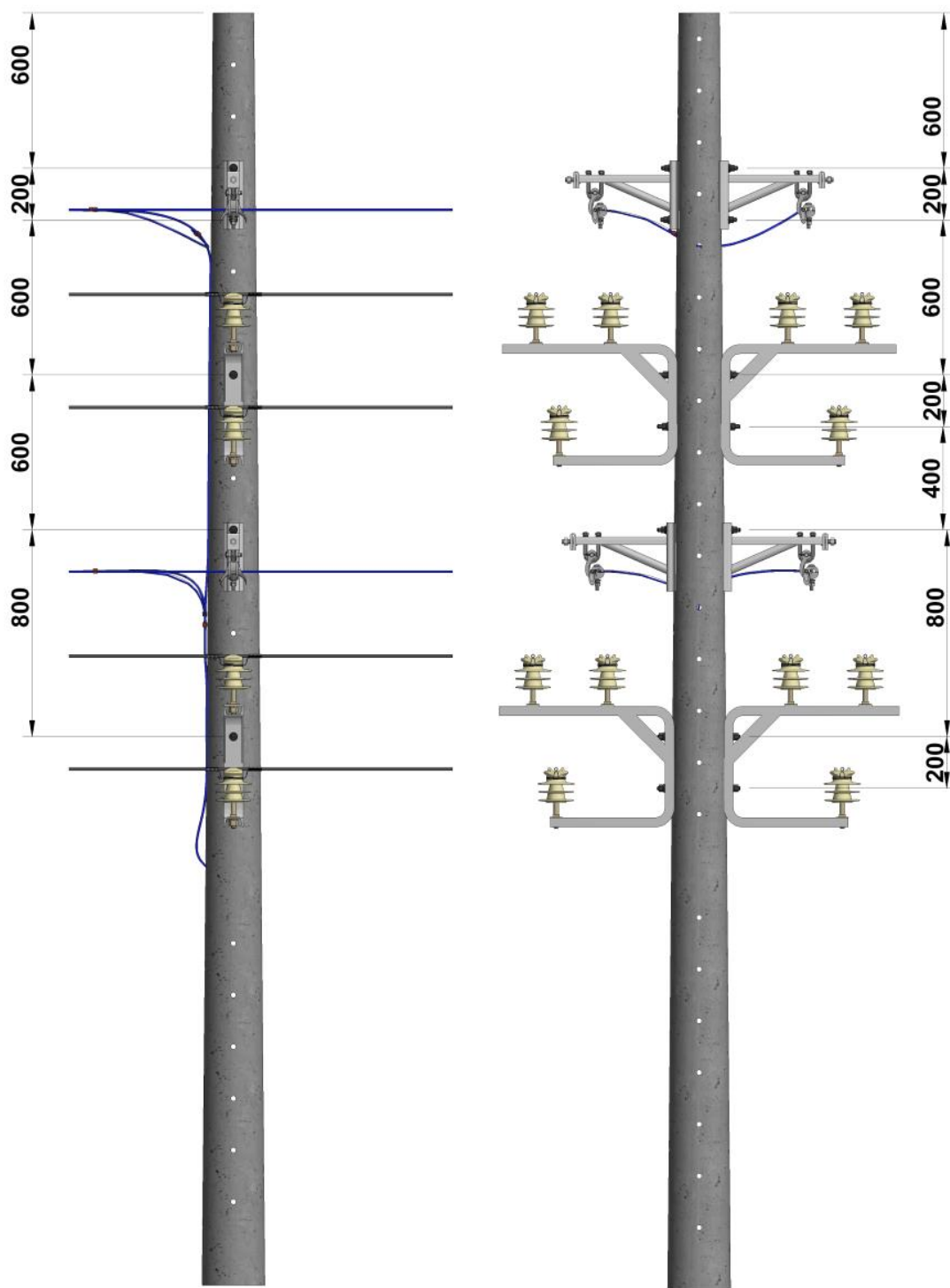
Figura 2. Vista frontal.
