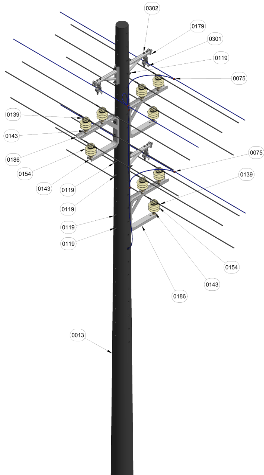
Figura 1. Vista isometrica.
