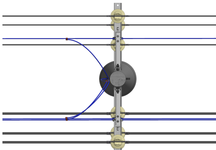
Figura 3. Vista en planta.
