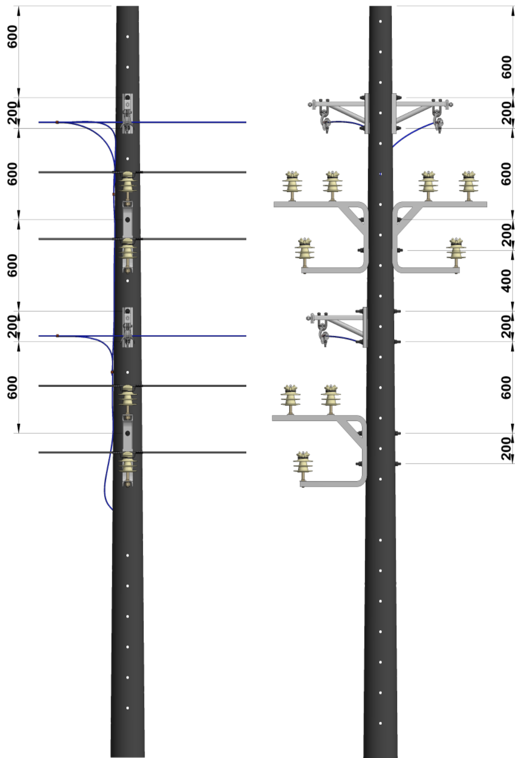
Figura 2. Vista frontal.
