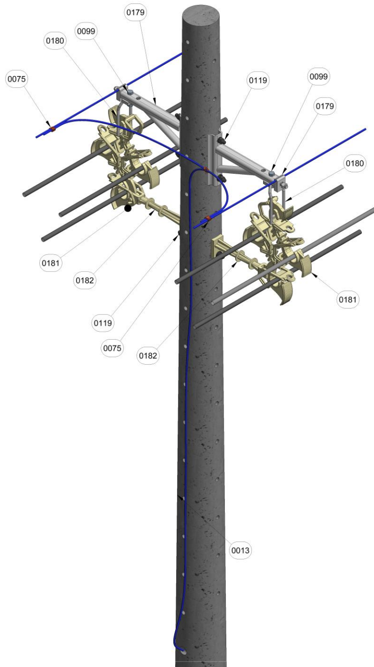
Figura 1. Vista isometrica.
