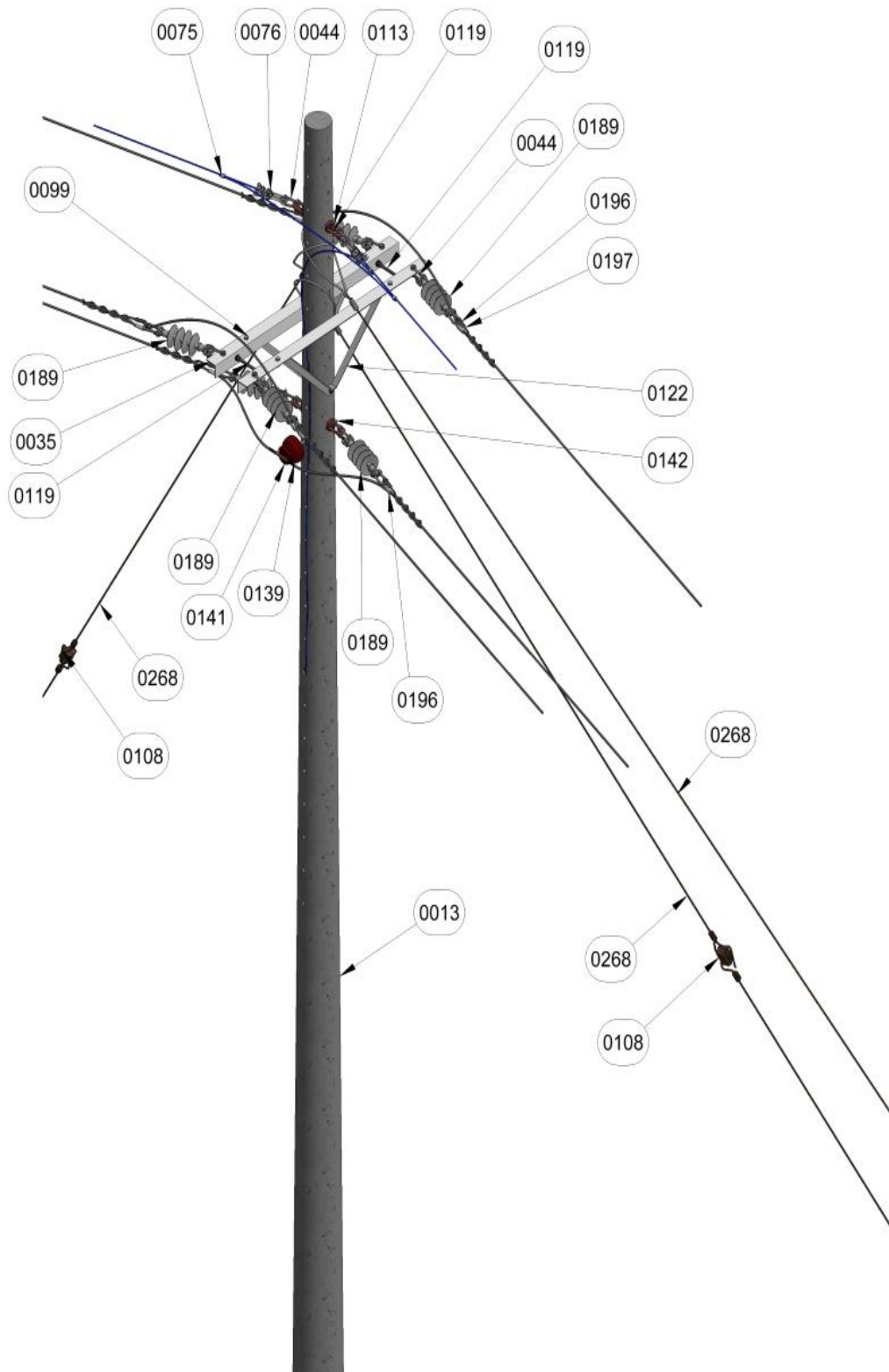
Figura 1. Vista isométrica.
