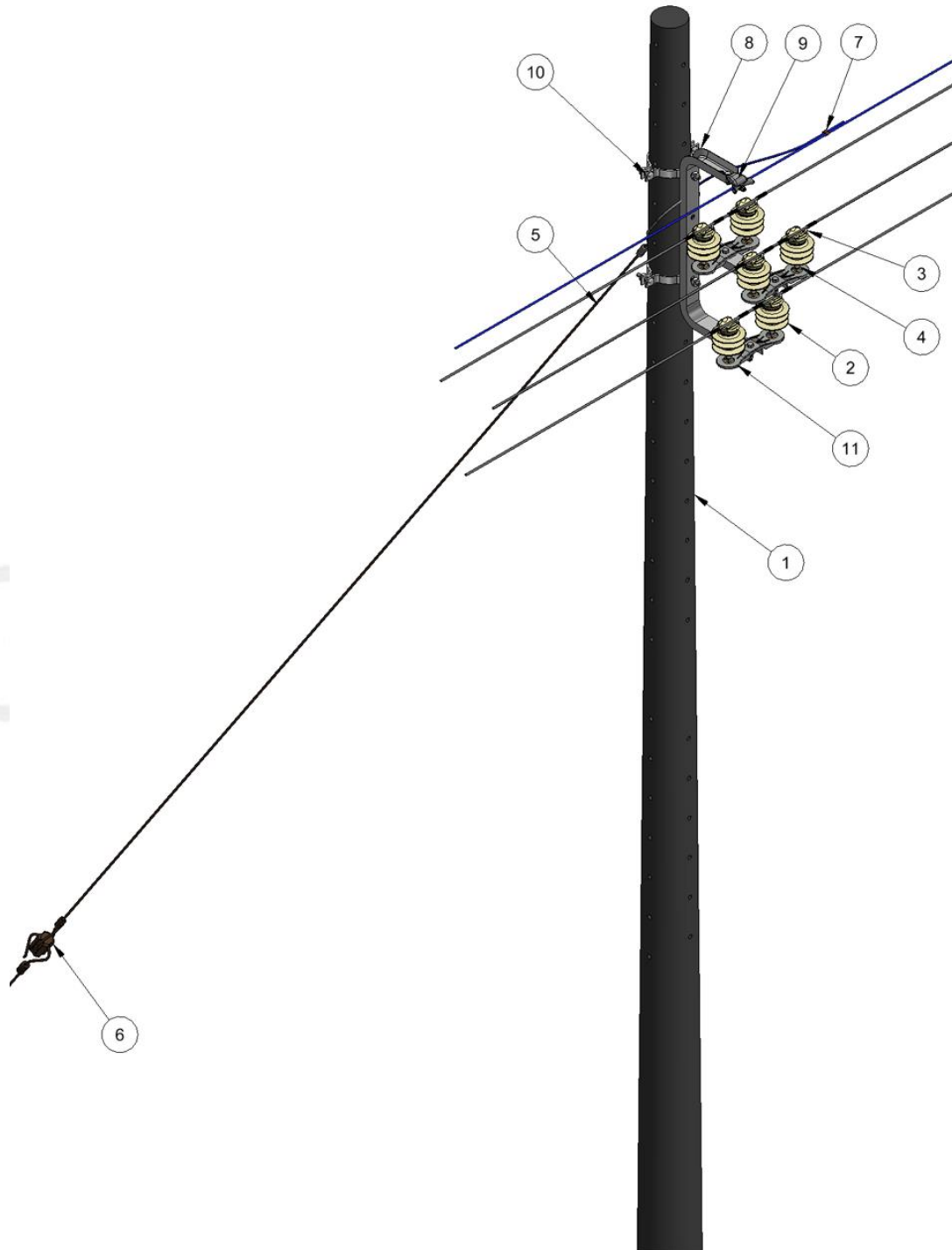
Figura 1. Vista isometrica.
