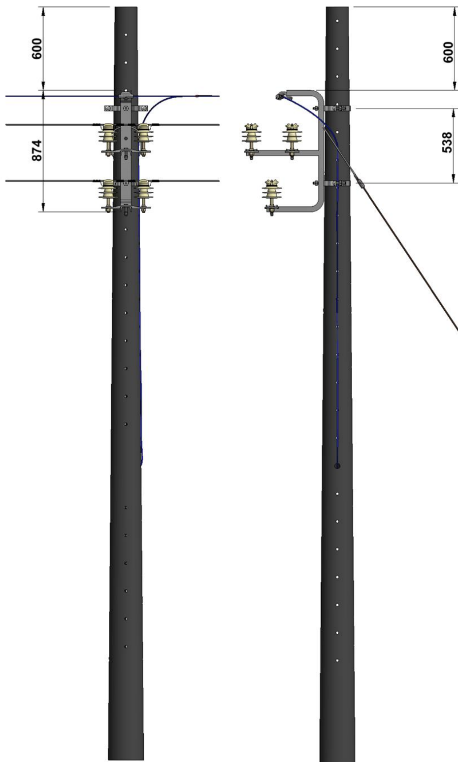
Figura 2. Vista frontal.
