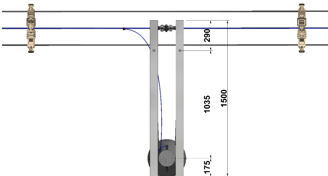
Figura 3. Vista en planta.
