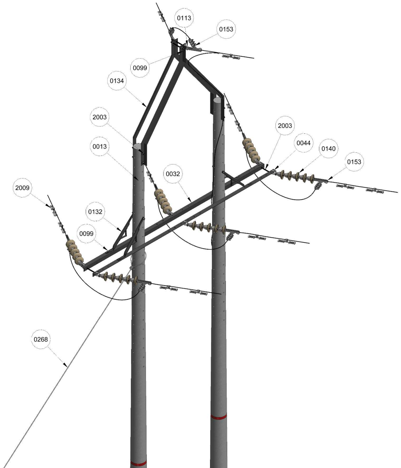
Figura 1. Vista isométrica
