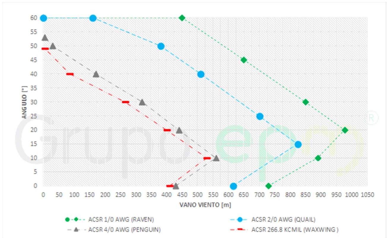
Figura 4. Curva de utilización para opción de montaje a: con retenida y sin bayoneta
