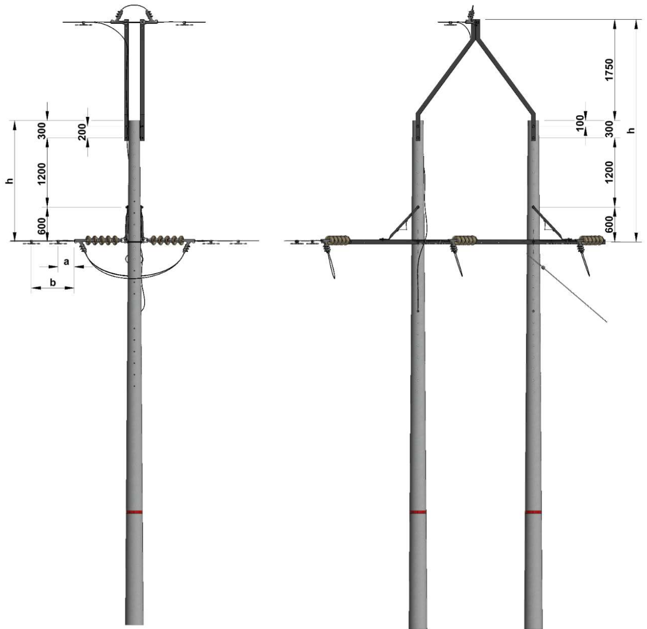
Figura 2. Vista frontal
