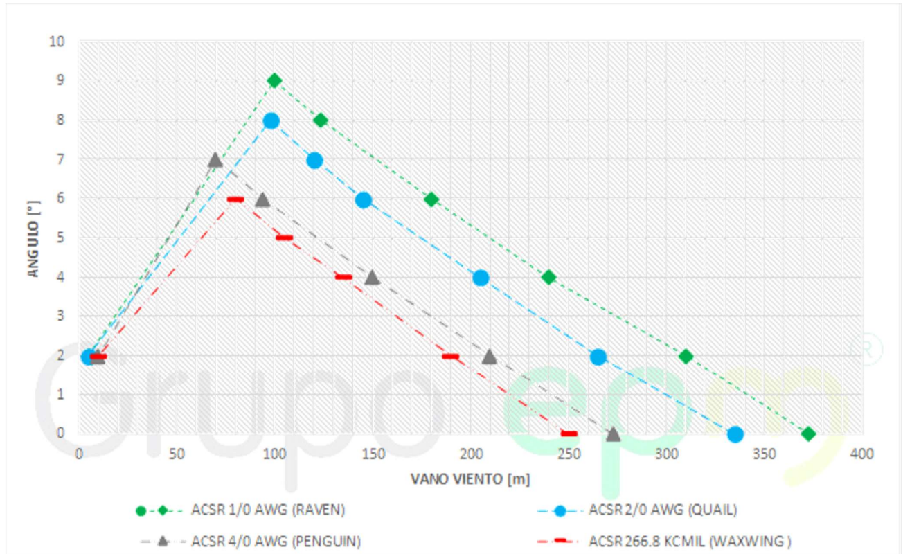
Figura 5. Curva de utilización para opción de montaje d: sin retenida y con bayoneta para soportar el cable de guarda
