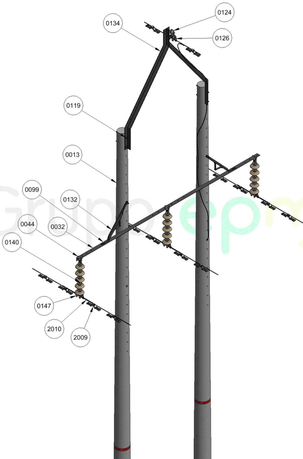
Figura 1. Vista isométrica
