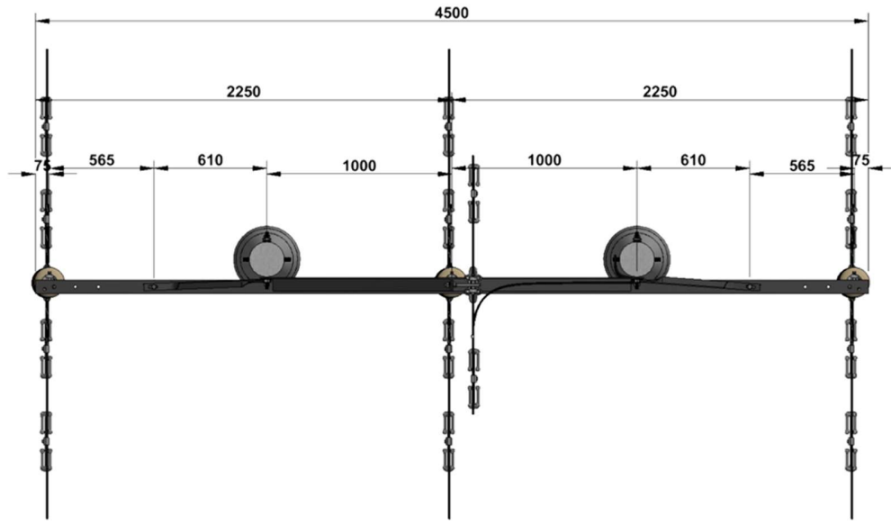
Figura 3. Vista en planta
