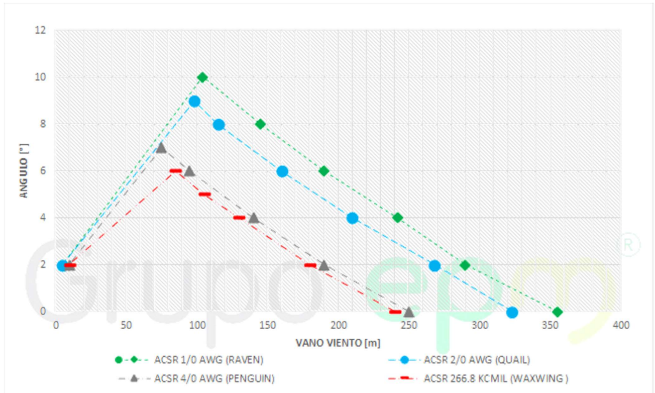
Figura 6. Curva de utilización para opción de montaje d: sin viento y con bayoneta o espigo para soportar el neutro
