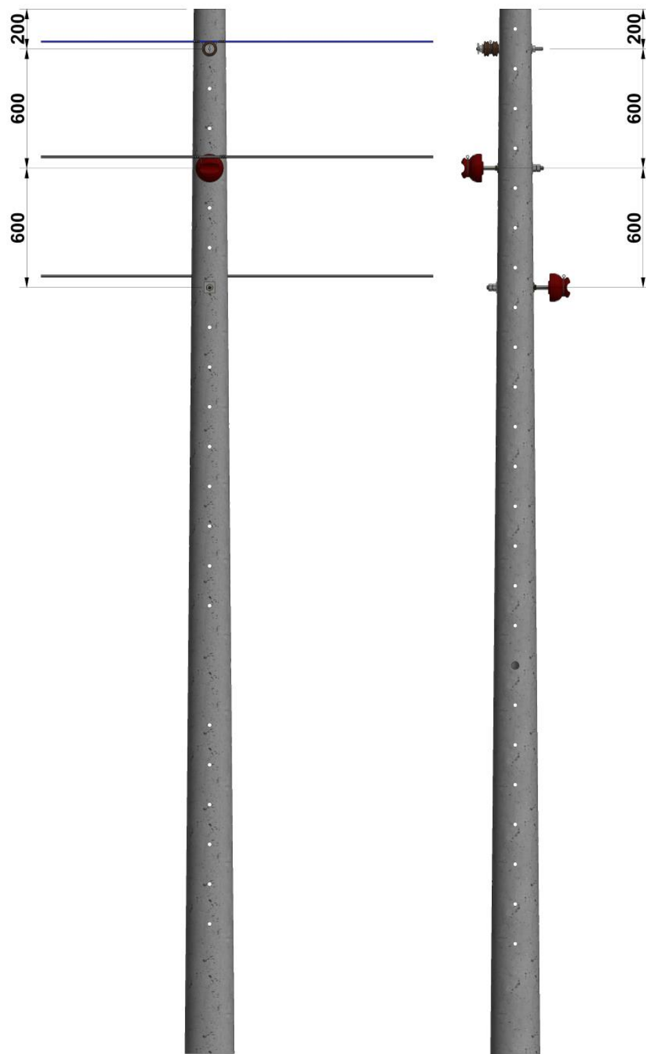
Figura 2. Vista frontal.
