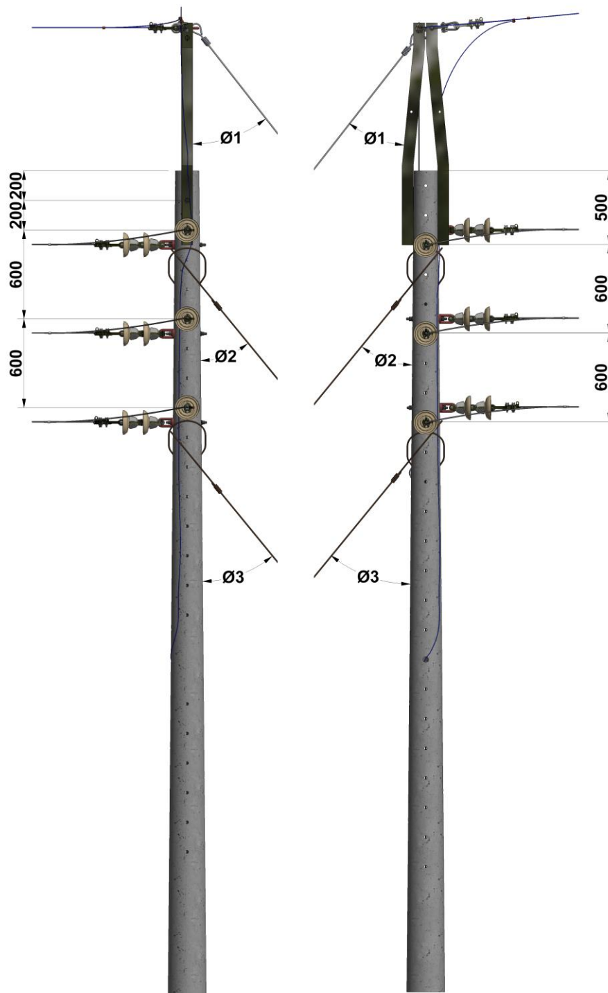
Figura 2. Vista frontal.
