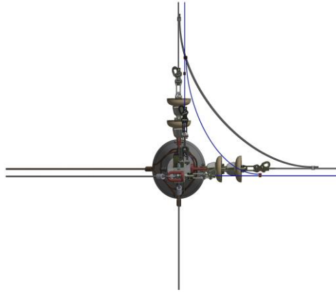
Figura 3. Vista en planta.
