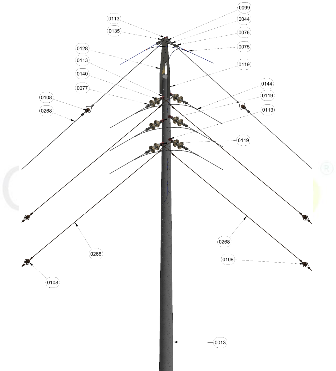
Figura 1. Vista isometrica.
