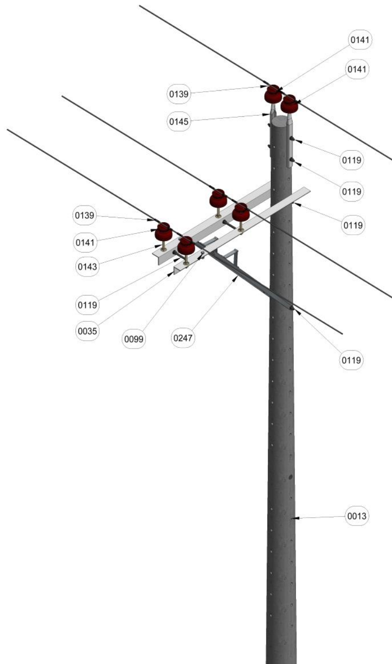
Figura 1. Vista isometrica.
