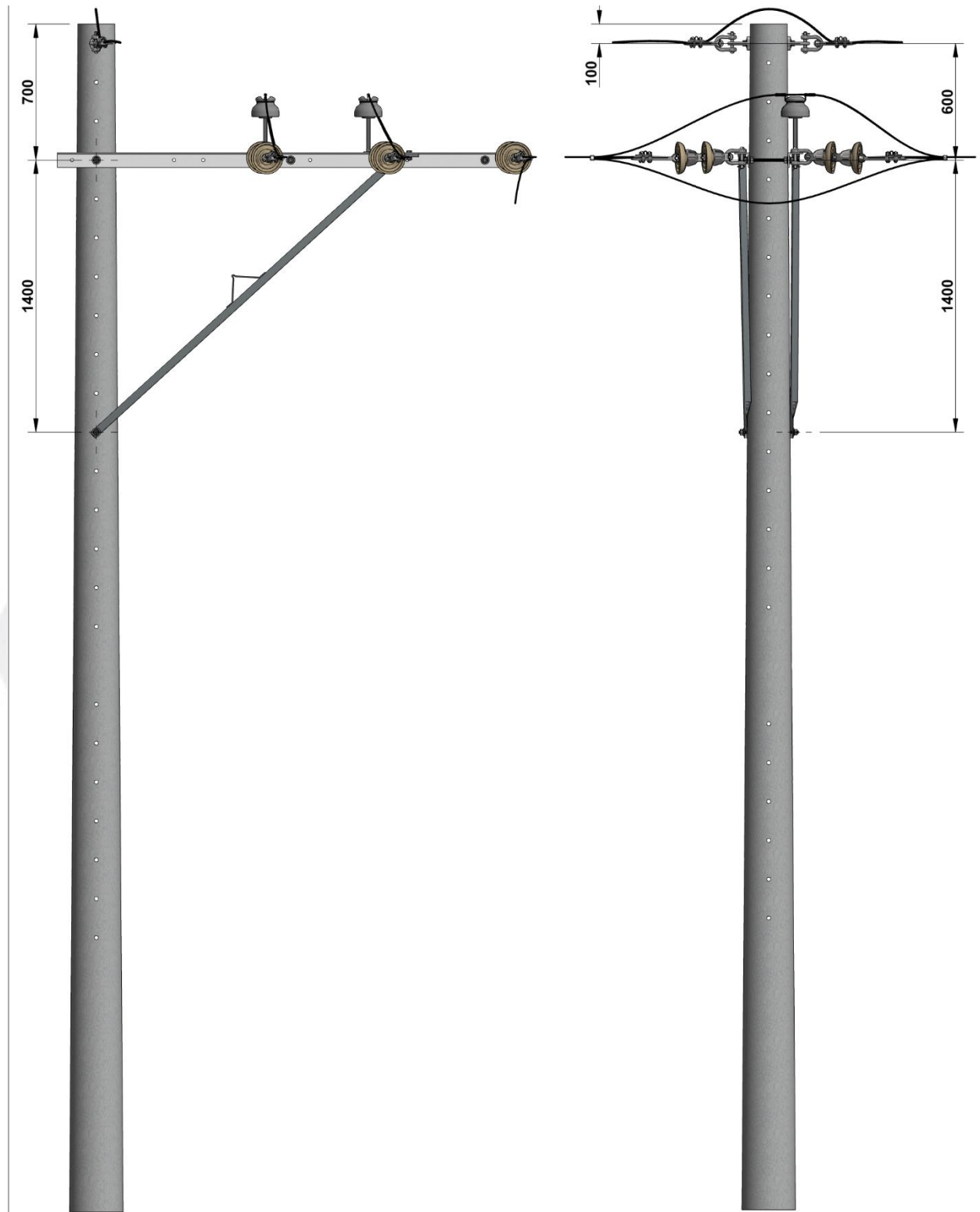
Figura 2. Vista frontal.
