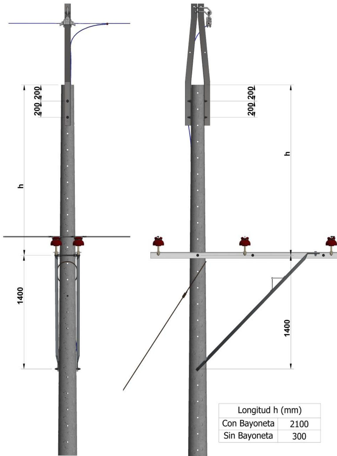
Figura 2. Vista frontal
