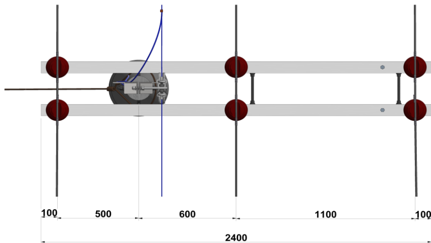
Figura 3. Vista en planta
