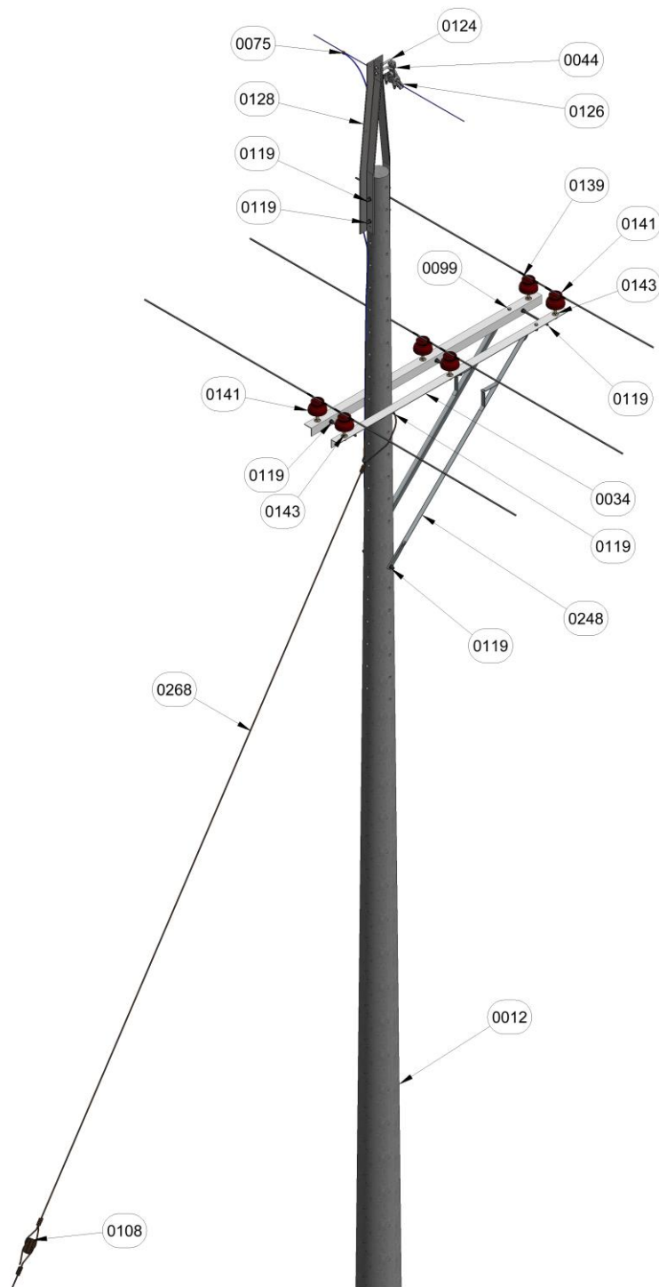
Figura 1. Vista isometrica
