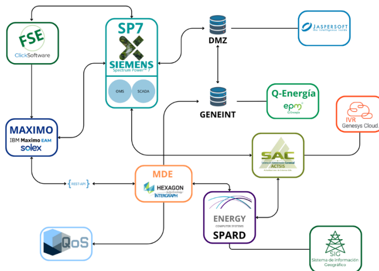
Figura 54. Esquema CENS Sistema de Gestión de Distribución
