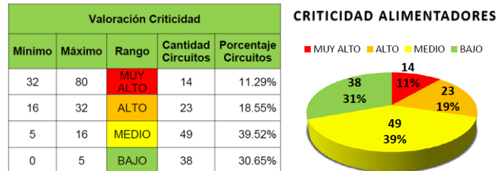
Figura 56. Criticidad Circuitos
