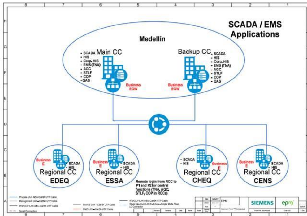
Figura 53. Funcionamiento SCADA Grupo EPM
