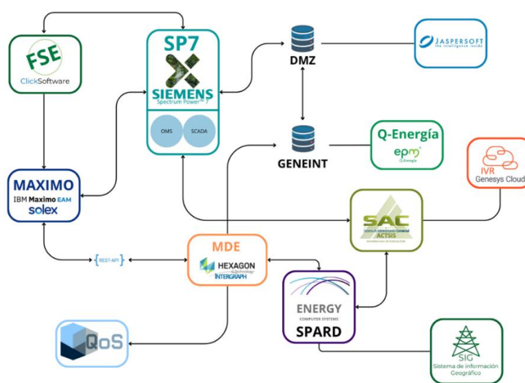
Figura 26. Esquema CENS Sistema de Gestión de Distribución
