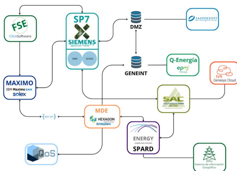
Figura 25. Esquema CENS Sistema de Gestión de Distribución
