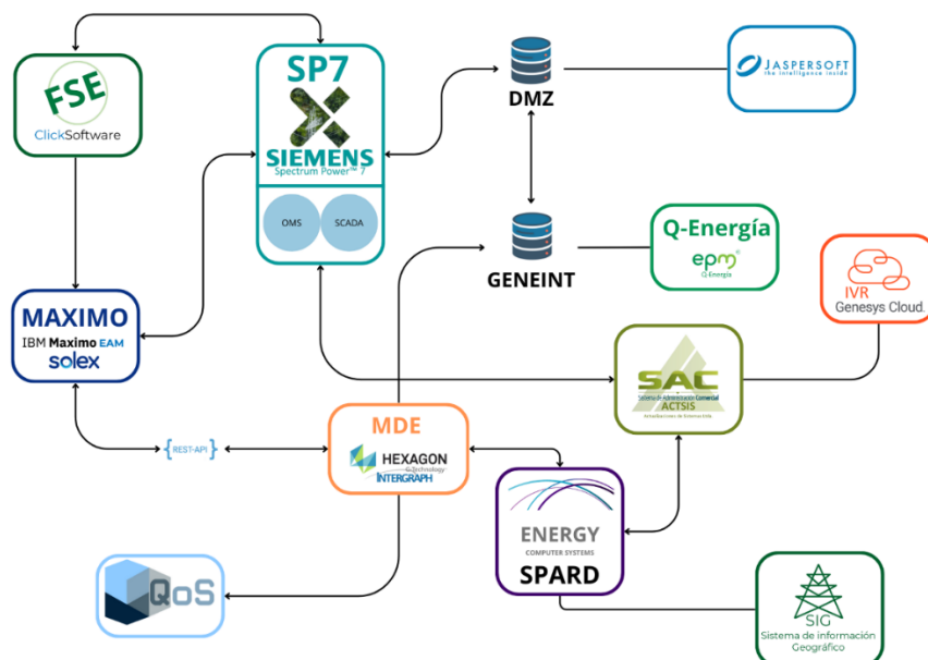
Figura 26. Esquema CENS Sistema de Gestión de Distribución
