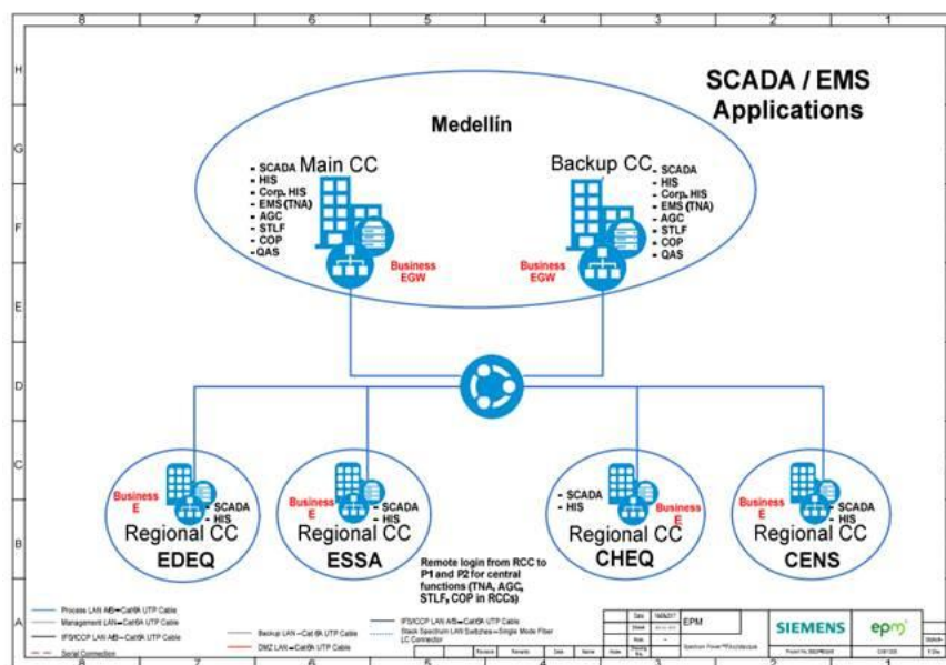
Figura 25. Funcionamiento SCADA Grupo EPM
