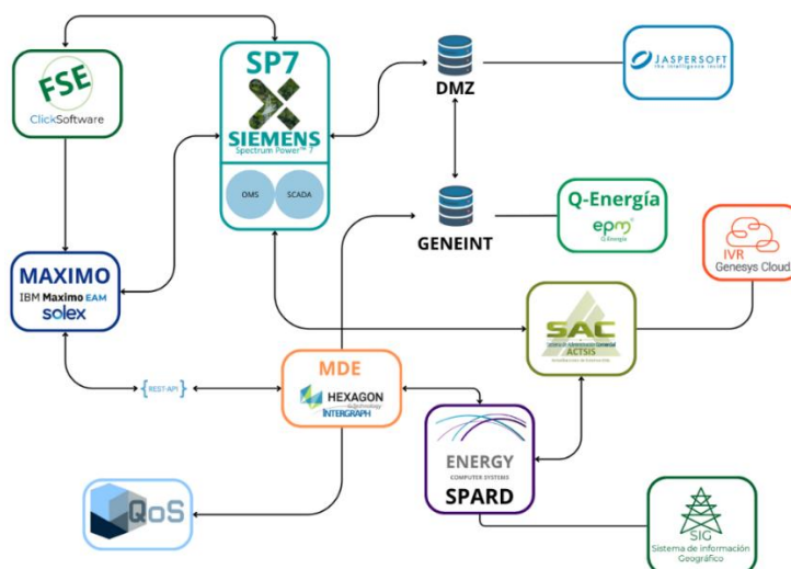
Figura 26. Esquema CENS Sistema de Gestión de Distribución
