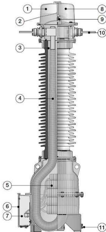
Figura 3. Transformador de corriente de uso exterior para media tensión Modelo IMB de ABB (ABB Power technologies, 2005)
