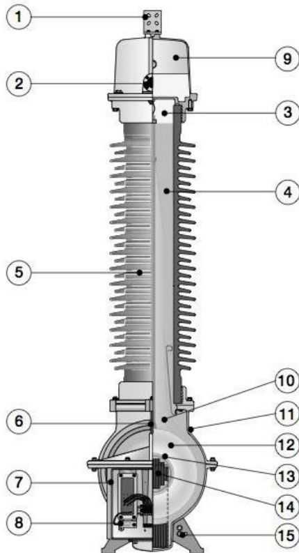
Figura 7. Transformador de tensión inductivo. Modelo EMF 14 de ABB (ABB Power technologies, 2005)
