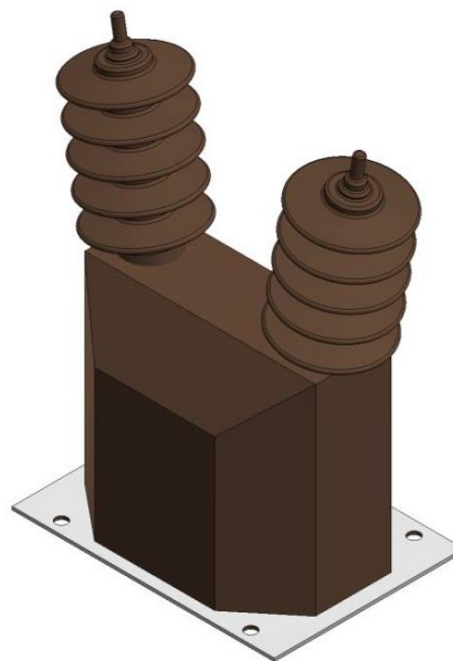
Figura 8. Modelo 3D de Transformador de tensión. Basado en Modelo VZF-36 de RITZ (RITZ Instrument Transformers)
