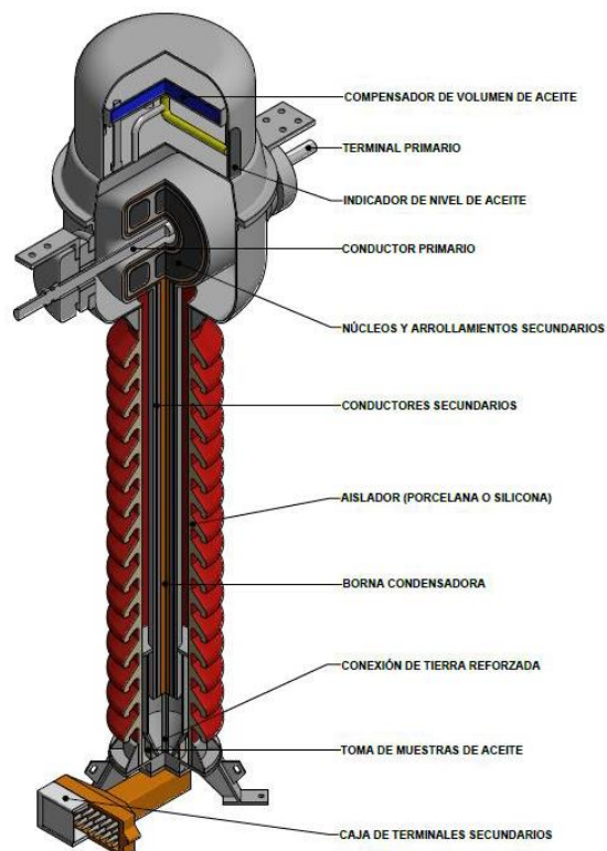
Figura 1. Modelo 3D de Transformador de corriente para alta tensión. Basado en el modelo CA del fabricante ARTECHE. (ARTECHE, ARTECHE - Catálogo Transformadores de Medida Alta Tensión. Versión B2)
