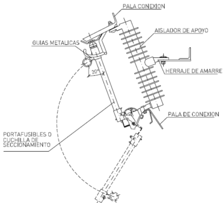
Figura 1: Esquema General del Cortacircuito.
